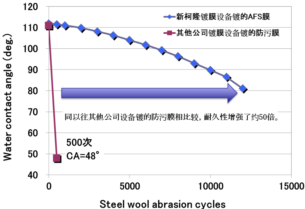
耐久性比较试验结果
